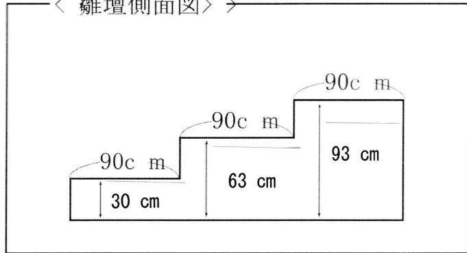
〈 雛壇側面図 〉
